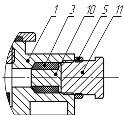
д) монтаж заглушки
