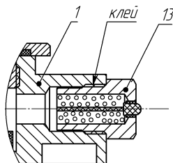
е) монтаж оконечного элемента
